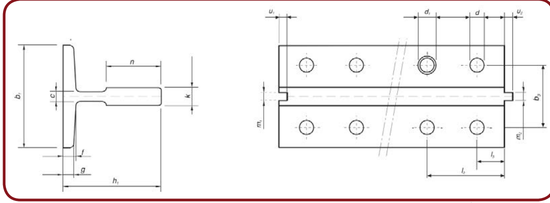
Fiziksel Ölçüler (mm) / Physical Dimensions (mm)
